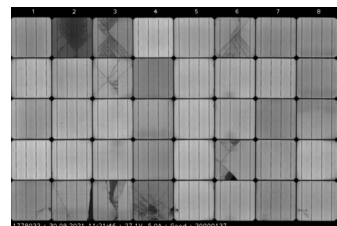
Abb. 6: Modul nach Hagel (Hagelkorngrösse: 6cm)
