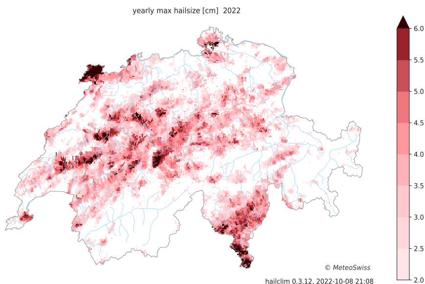
Abb 1: MeteoSchweiz, Hagelkarte 2022 - maximale Hagelkorngrösse
