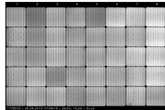
Abb. 5: Modul bei Auslieferung
