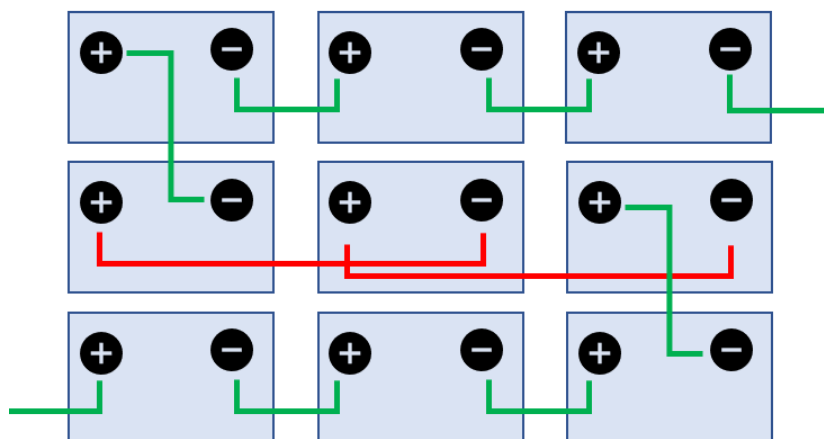
Abb. 3: Verschaltungsskizze
